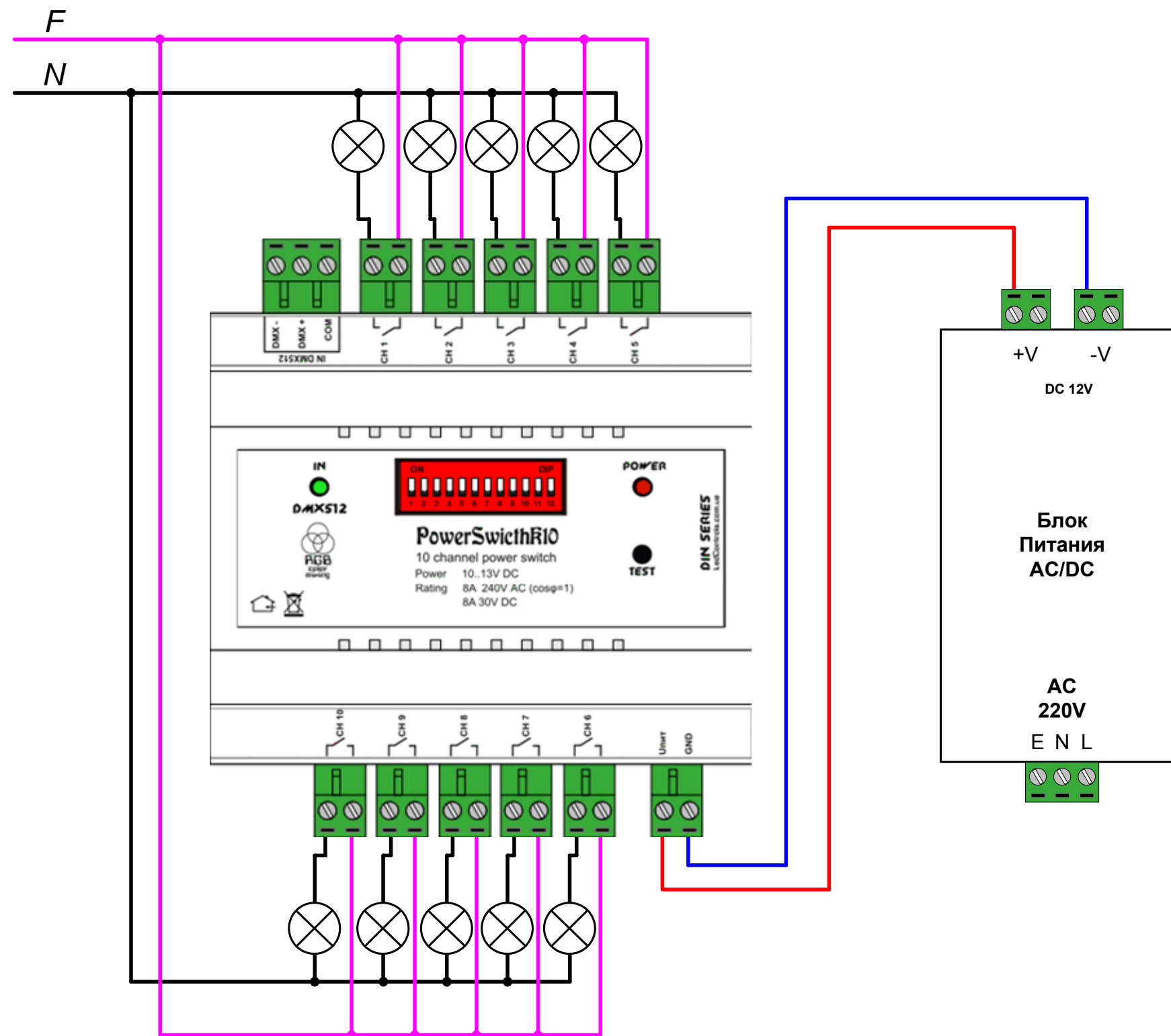
Схема подключения нагрузки с напряжением питания 220V AC.
